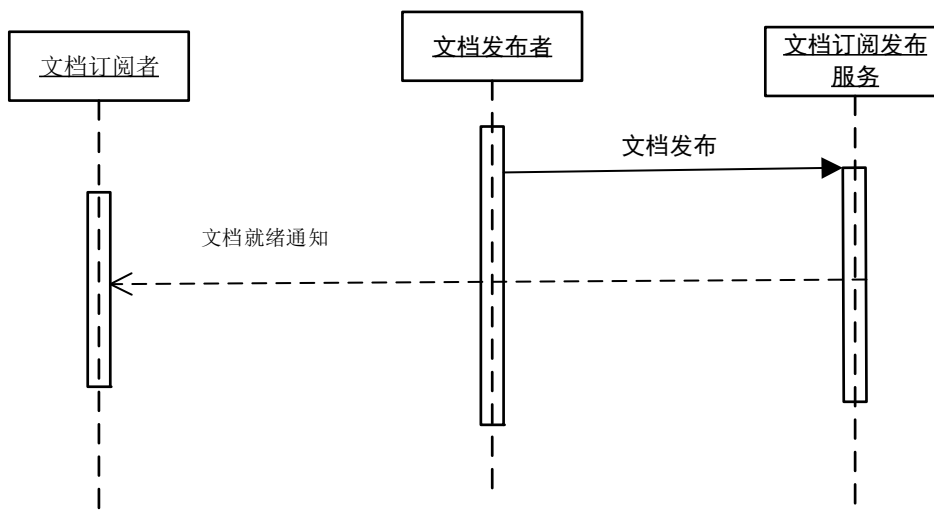
图11 文档发布与就绪通知交易流程图
